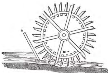
Strømhjul, skematisk (Efter J. Witckens)
