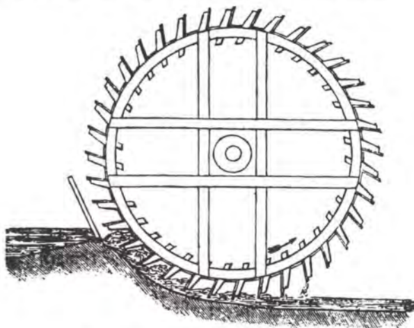
Underfaldshjul, skematisk (Efter J. Witckens)
