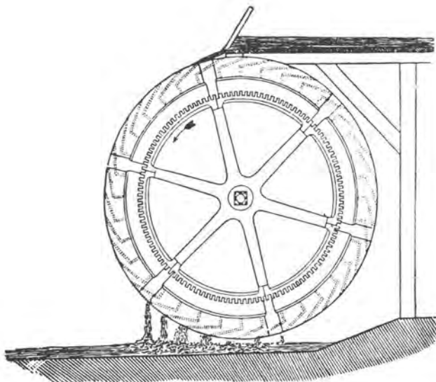
Overfaldshjul, skematisk (Efter J. Wilckens)
